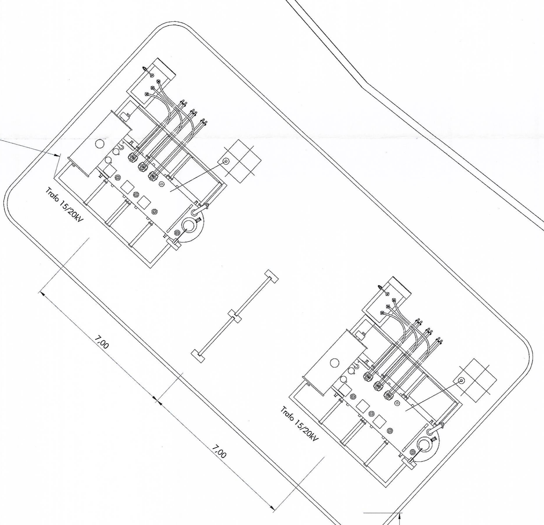
Planimetrie piazzale scala 1:100
