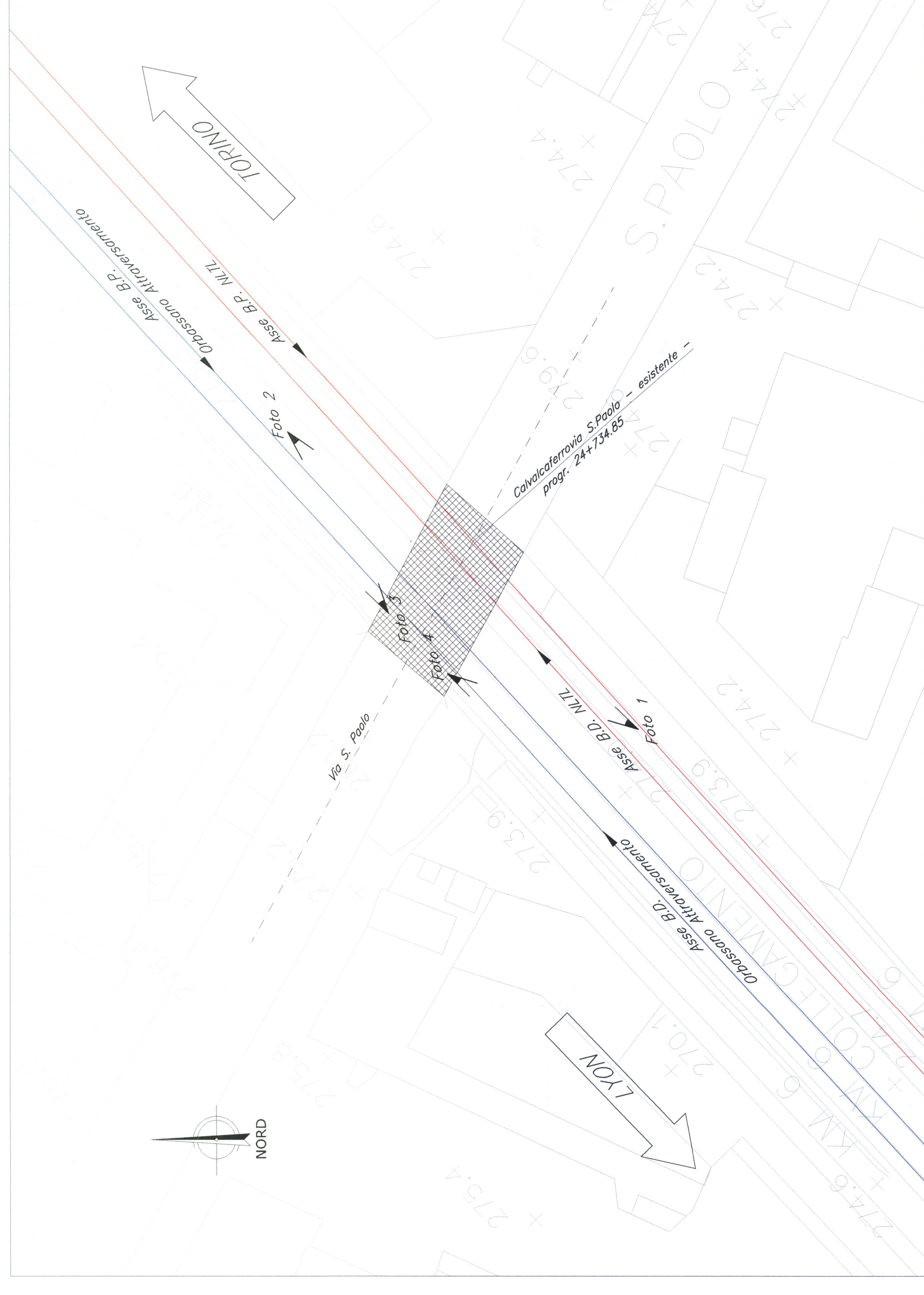
Stralcio planimetrico
