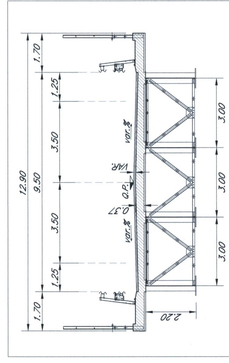
Sezione stradale Tipo C2
