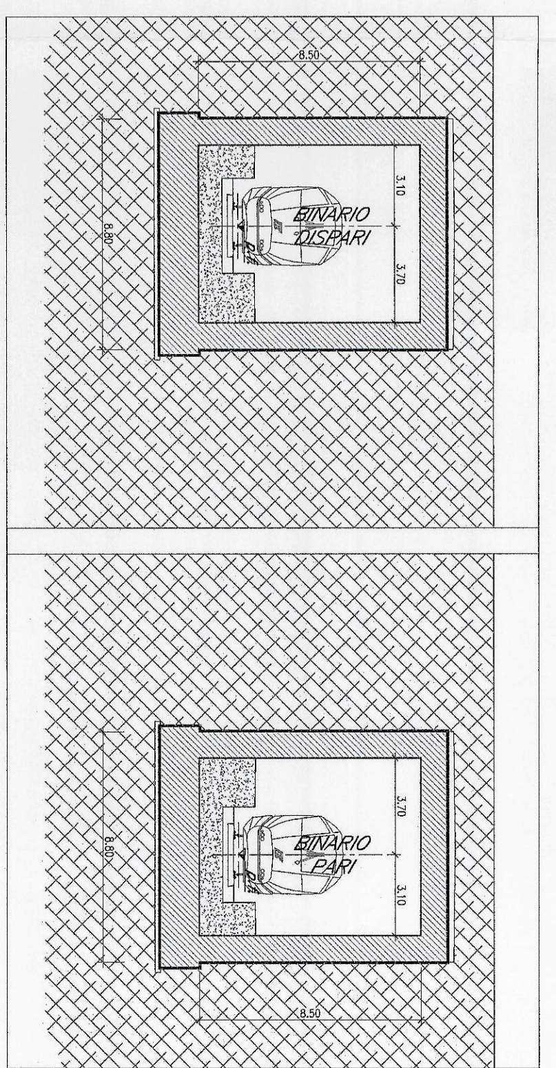
SEZIONE TIPO CORRENTE - Scala 1:200 -
