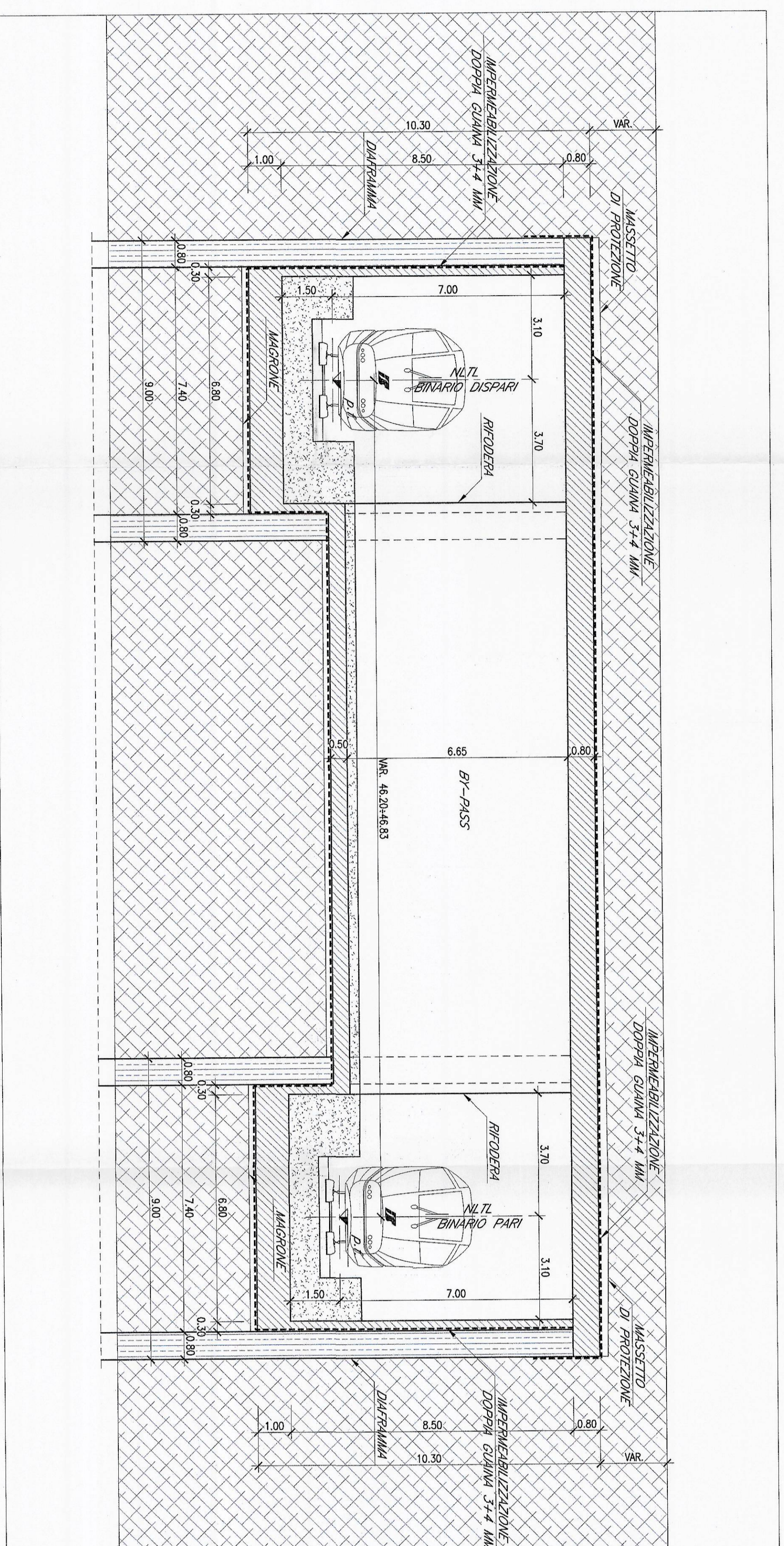
SEZIONE TRASVERSALE TIPO in corrispondenza dei BY-PASS — Scala 1:100 —
