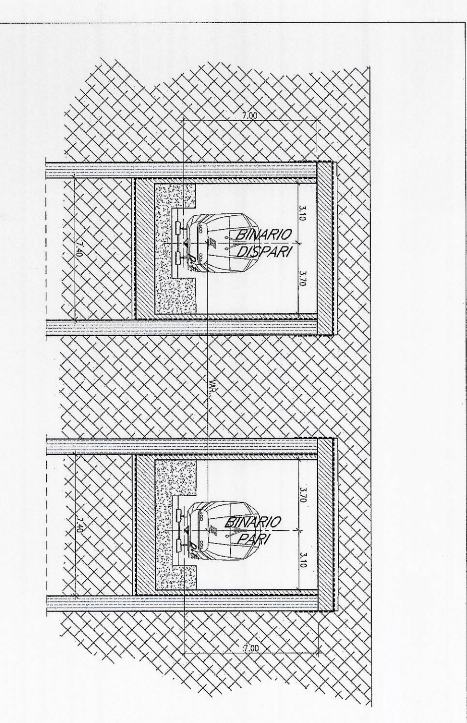
SEZIONE TIPO CORENTE - Scala 1:200 -
