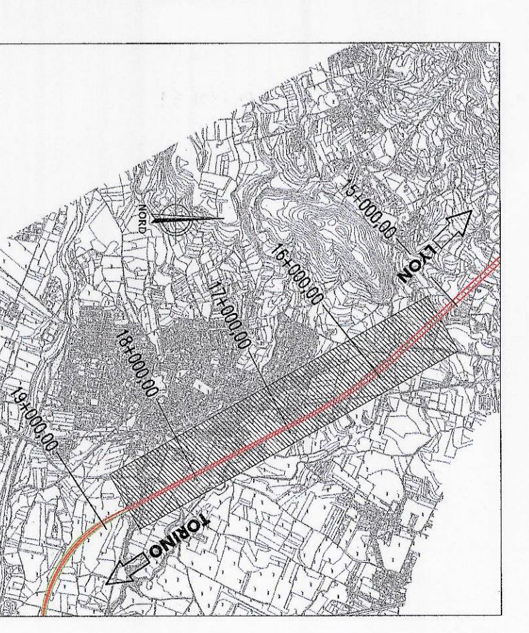
PIANTA CHIARE
